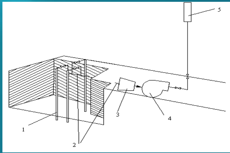
сбор биогаза
